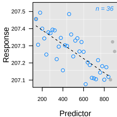
-- : L_{pc} Rank 1: y = 207.47 - 0.0004 \cdot x
