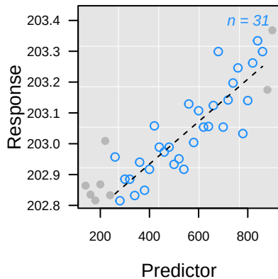
-- L_{pc} Rank 1: y = 202.66 + 0.0007 \cdot x
