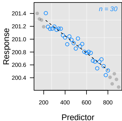
-- L_{pc} Rank 1: y = 201.59 - 0.0013 \cdot x
