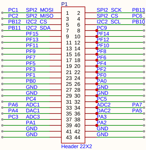
扩展接口,焊接排针在底面
