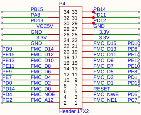
LCD屏幕,焊接排母在表面
