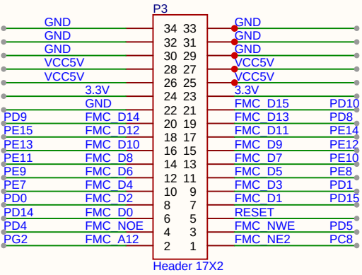
FPGA接口,焊接排针在底面
