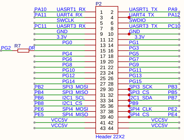
扩展接口,焊接排针在底面
