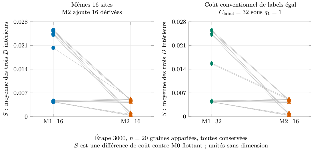
Figure 2: Vingt paires à 3000, toutes conservées. Une liaison représente une graine. À gauche : mêmes sites et dérivées supplémentaires ; à droite : coût de labels égal uniquement sous q_1 = 1 . Provenance : F2.
