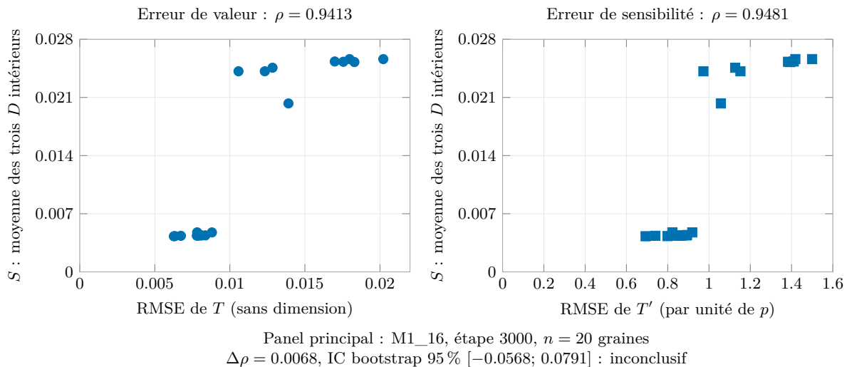
Figure 4: Panel principal à 3000, n = 20 . Même échelle verticale dans les deux panneaux. Aucune régression ou combinaison avec les panels secondaires. Provenance : F4.
