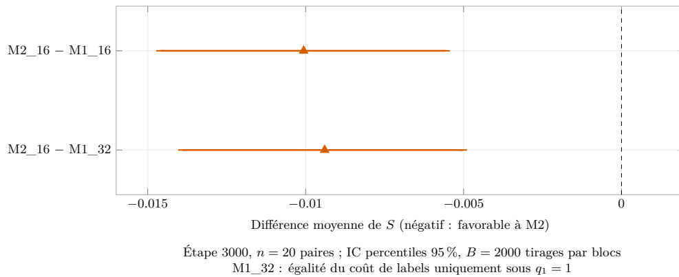
Figure 3: Différences moyennes de S et IC bootstrap percentiles à 95 %, B = 2000 , n = 20 graines. Le signe négatif favorise M2. Provenance : F3.
