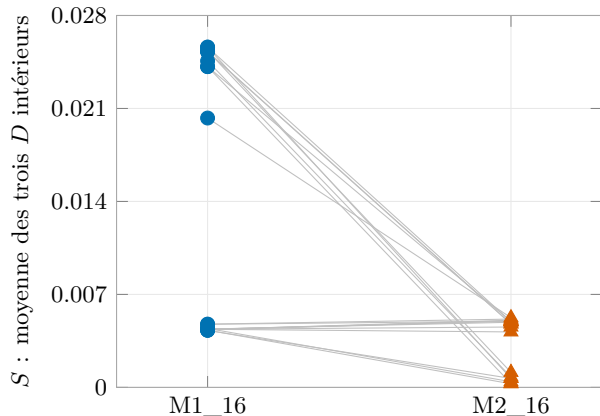
Mêmes 16 sites M2 ajoute 16 dérivées
