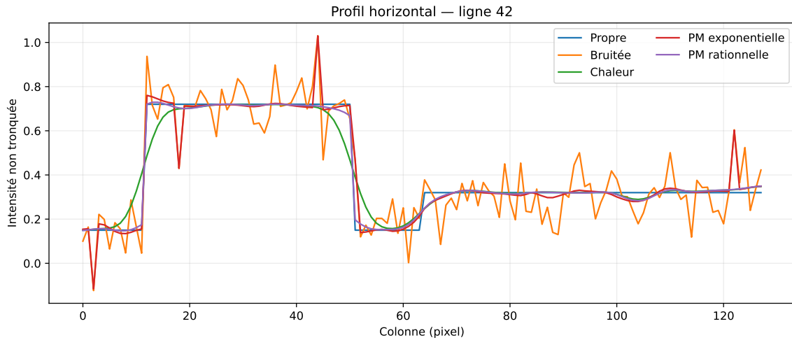
Figure 5.2: Profil horizontal, ligne 42, du même cas individuel geometric_shapes , \sigma = 0,10 , graine 0, n = 20 , t = 4 , K = 0,10 , \Delta x = \Delta y = 1 , \Delta t = 0,20 . Intensités non tronquées : élargissement des transitions par la chaleur et pics résiduels de la PM exponentielle. Il ne s'agit pas d'une moyenne sur les graines.
