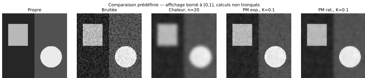
Figure 5.1: Cas individuel préfixé : geometric_shapes , \sigma = 0,10 , graine 0, n = 20 , t = 4 ; K = 0,10 pour les deux PM, \Delta x = \Delta y = 1 , \Delta t = 0,20 . Échelle d'affichage commune [0, 1] , sans troncature des tableaux évalués. L'exponentielle conserve ici des fluctuations que la rationnelle atténue davantage ; aucune bande statistique.
