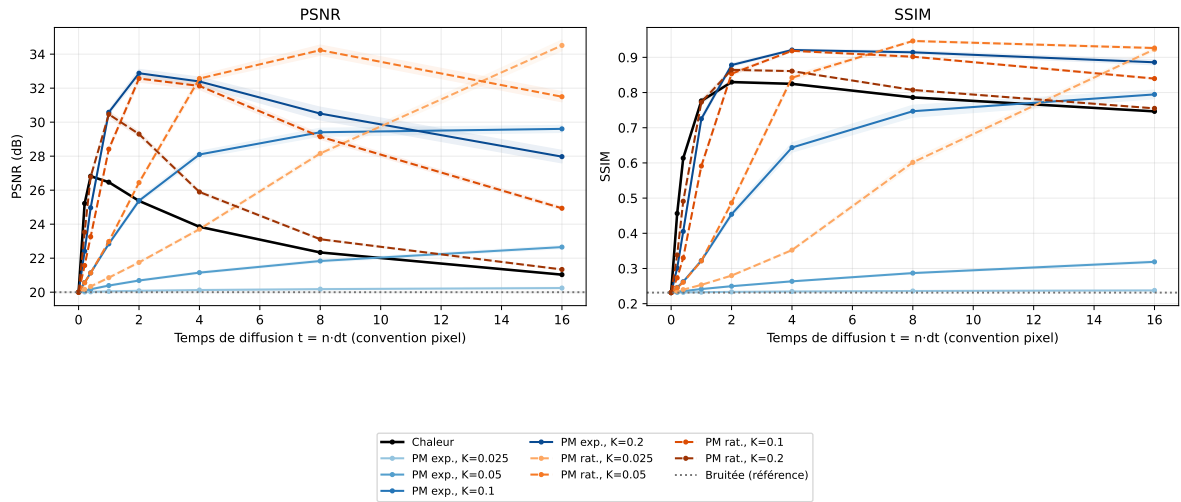
Figure 5.6: PSNR et SSIM agrégés pour \sigma = 0,10 : geometric_shapes en haut, ramps_and_edges en bas. Moyennes et bandes \pm un écart-type échantillonnel sur dix graines. Chaleur et huit PM avec K = 0,025; 0,05; 0,10; 0,20 ; \Delta x = \Delta y = 1 , \Delta t = 0,20 , huit checkpoints jusqu'à t = 16 . Les petits K exponentiels conservent du bruit ; la poursuite des variantes plus diffusives peut conduire au sur-lissage.
