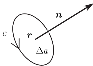
図 10.16 右ネジの規則
