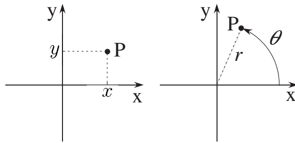
図 6.1 二次元平面のデカルト座標 (左) と極座標 (右)。デカルト座標では、点 P から二つの軸におろした垂線から座標の値 x, y を決める。極座標では、点 P と原点との距離を r とし、P と原点を結ぶ線分と x-軸のなす角を \theta とする。
