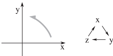
図 10.15 「正の回転の向き」の規則。xy 面内での正の向きの回転とは、左図のように、x 軸正の側から y 軸正の側にむかう回転をいう。同様に、yz 面内では、y 軸正から z 軸正が正の回転、zx 面内では、z 軸正から x 軸正が正の回転である。x, y, z の三つの座標の関係は、右図のような「三棘み (じゃんけんと同じ関係)」になっている (6.2.1 節を参照)。
