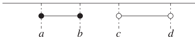
図 2.6 数直線上に、実数 a < b < c < d に対応する点を示す。下は、閉区間 [a, b] と開区間 (c, d) 。黒丸の点は区間に含まれ、白抜きの点は区間に含まれない。
