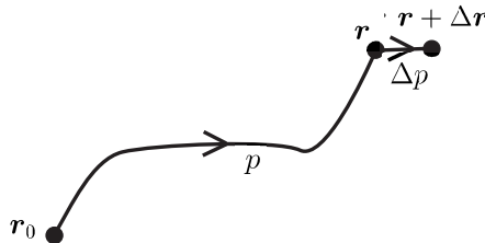
図 10.14 基準点 \mathbf{r}_0 から \mathbf{r} + \Delta \mathbf{r} へ向かう道 p' として、いったん \mathbf{r} を通過してから、まっすぐに \mathbf{r} + \Delta \mathbf{r} に向かうものを選ぶ。
