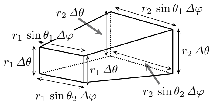
図 10.37 \Delta r , \Delta\theta , \Delta\varphi が小さいときの、立体図形 D の各辺の長さ。ただし、 r_1 = r - \Delta r/2 , r_2 = r + \Delta r/2 , \theta_1 = \theta - \Delta\theta/2 , \theta_2 = \theta + \Delta\theta/2 と書いた。図に記入していない「奥行き」の四本の線の長さはいずれも \Delta r である。このように形が「いびつ」であるため、互いに向き合っている、面 adhe と面 bcbf 、また、面 abcd と面 efgh の面積が等しくならない（面 abfe と面 dcgh の面積は等しい）。これが、ダイバージェンスの表式 (10.9.18) が複雑な理由である。
