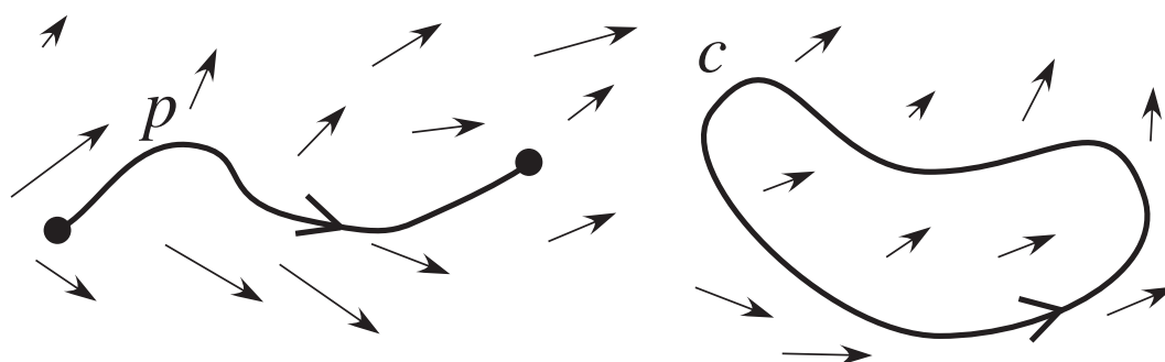
図 10.5 ベクトル場と、その中の二つの向きのついた道 p と c 。左側の道 p には始点と終点がある。右側の c は「閉じた道」であり、終わりの始まりもない「輪っか」になっている。これは、 p のような道で、たまたま始点と終点一致したものと思ってもよい。
