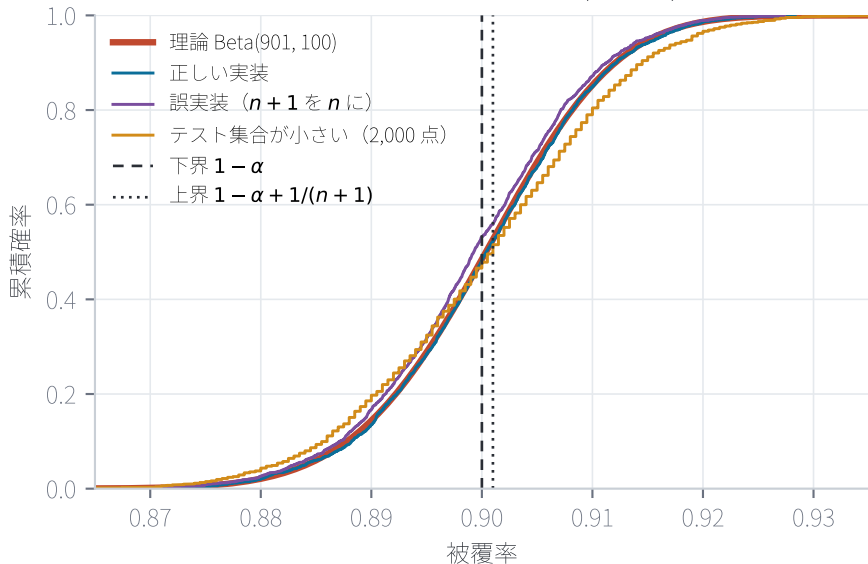
E1b：被覆率の経験分布関数 ( n = 1000, \alpha = 0.1, 2000 試行)
