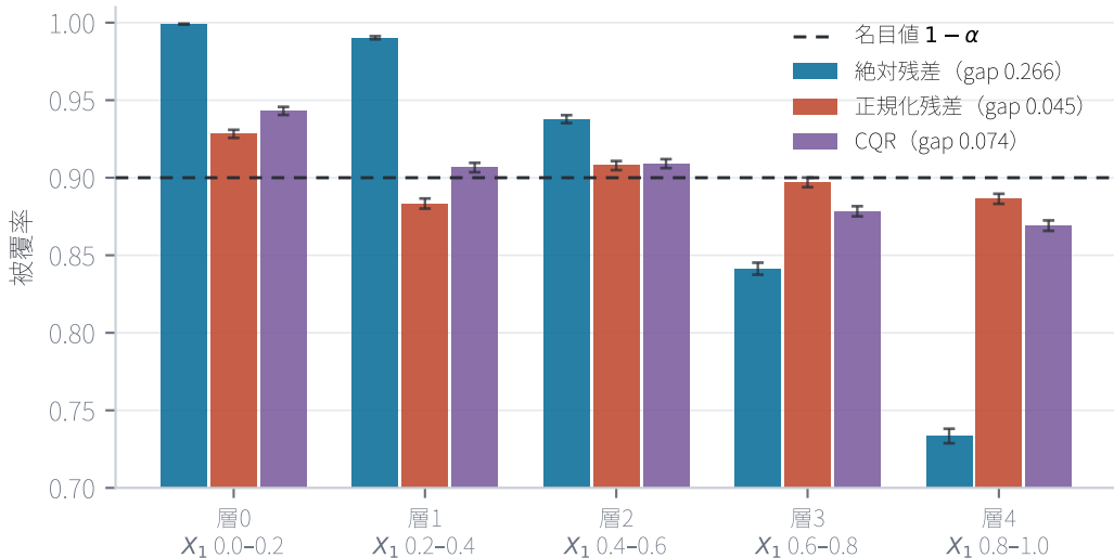
X_1 で層別した被覆率（誤差棒は試行間+テスト集合間 95%）
