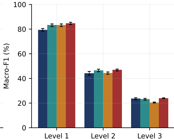
Macro-F1
