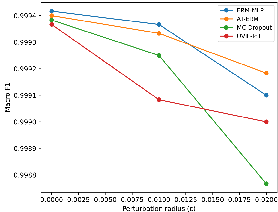
PGD Robustness — NBAIOT
