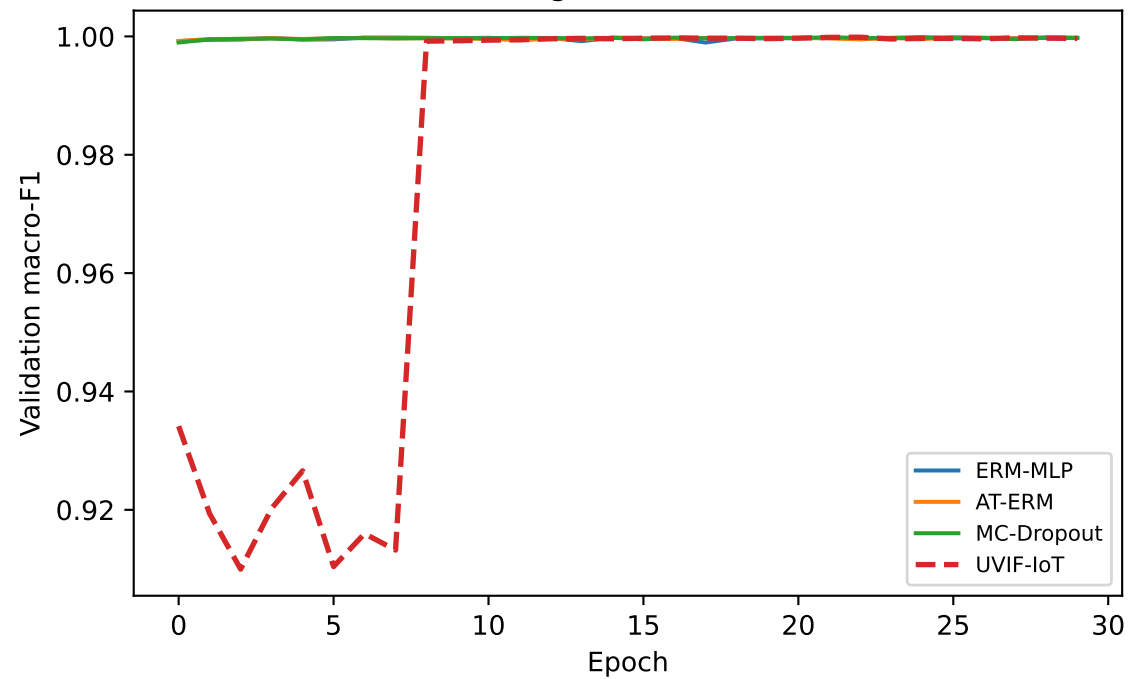
Convergence — NBAIoT
