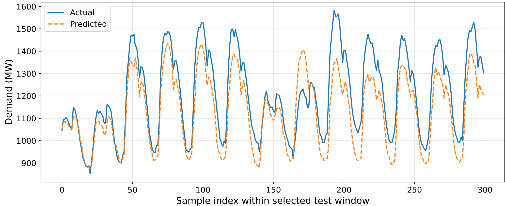
Electricity demand: Actual vs Predicted (first 300)
