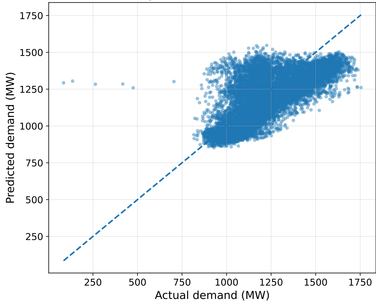
Electricity demand: Actual vs Predicted
