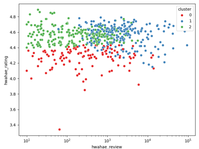
[그림 4] K-Means 군집 결과
