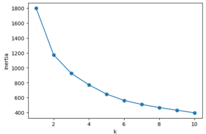
[그림 3] Elbow Method 결과
