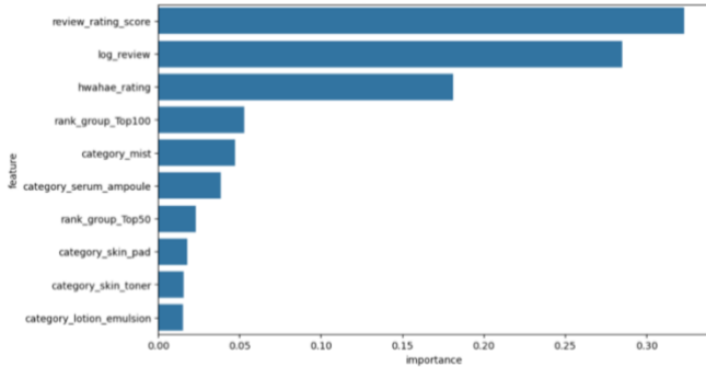
[그림 2] 변수 중요도(Feature Importance)
