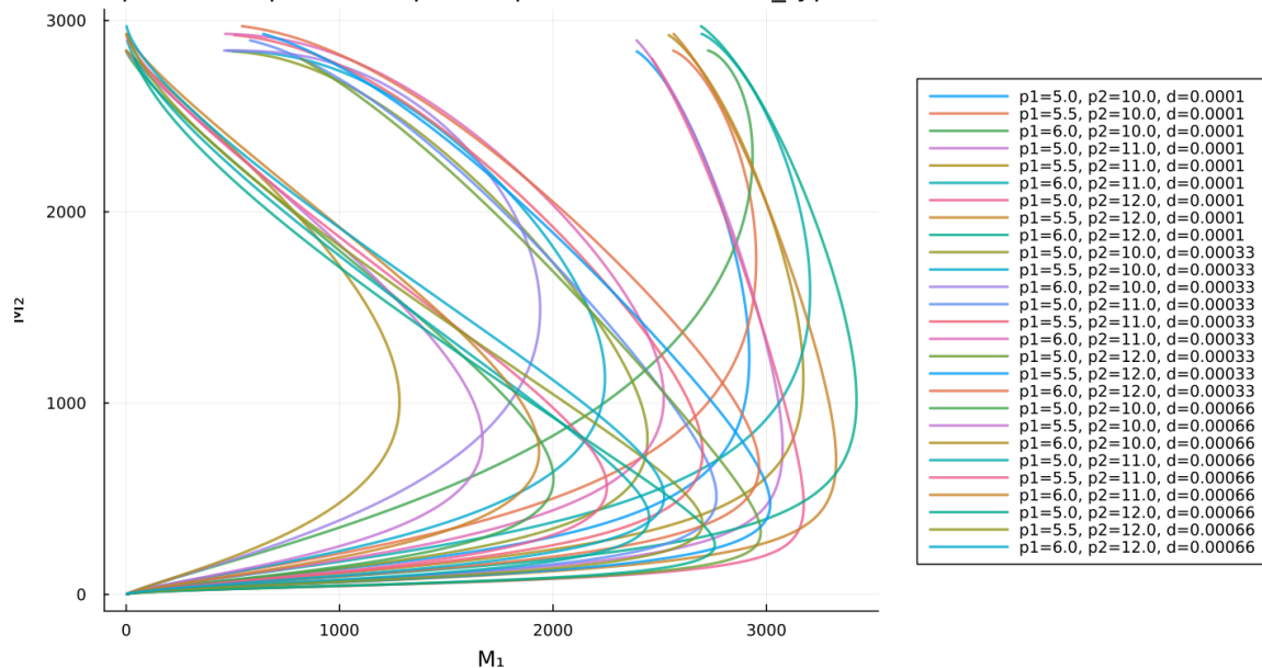
Рисунок 5.16: Сканирование: фазовые траектории M_2(M_1) , вторая модель
