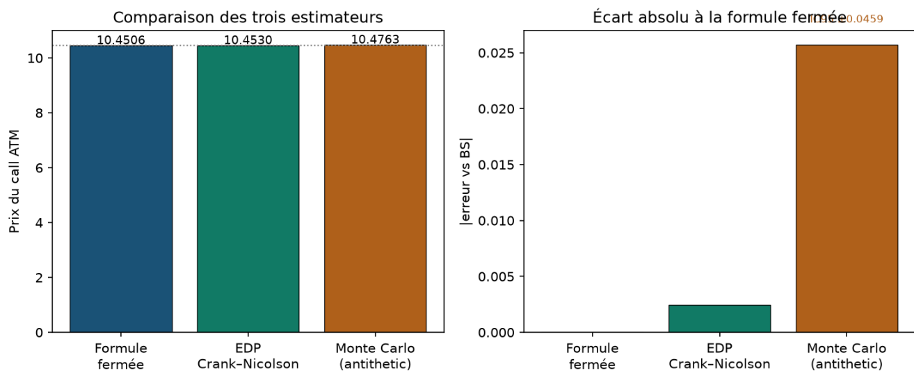
Figure 10: Figure 10 — Comparaison des méthodes
