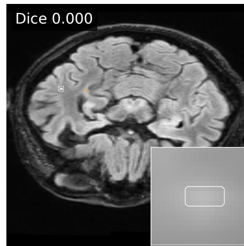
U-Net
