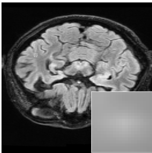
Input FLAIR
