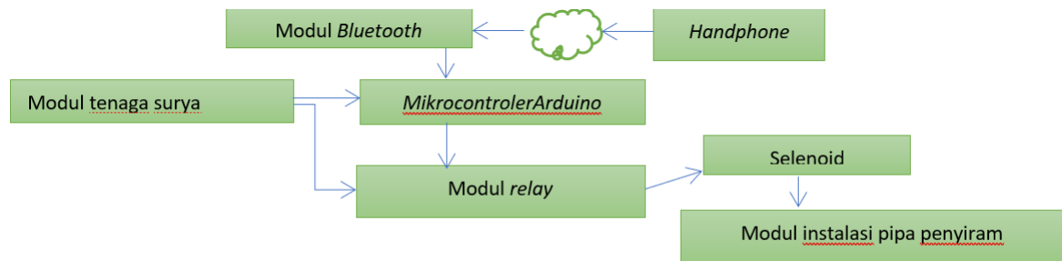
Gambar 1. Blok Diagram Alat yang dibuat
