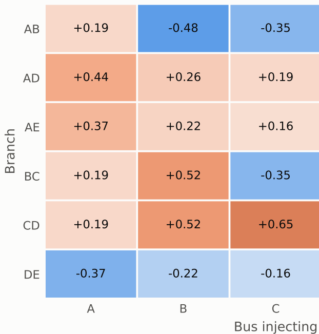
(a) Shift factors, slack D (MW/MW)
