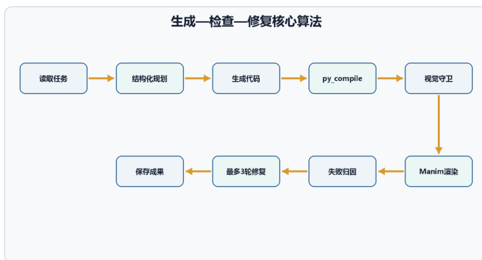
图 5-2 生成、检查、渲染和修复算法
