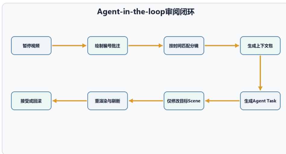
图 5-3 交互批注到局部修订的闭环
