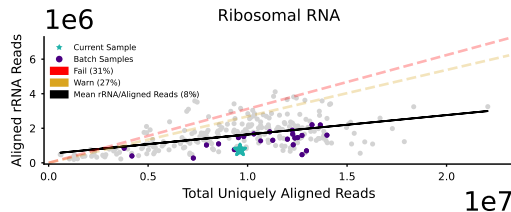
Ribosomal RNA
