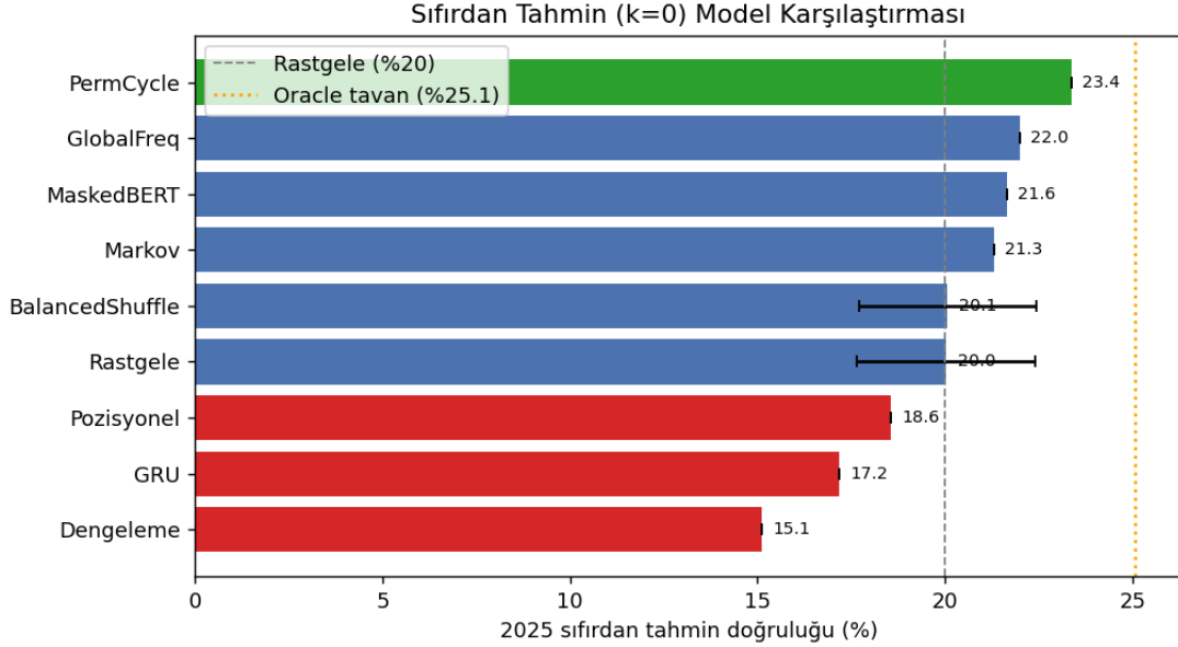
Şekil 2: Sıfırdan tahmin model karşılaştırması. Yeşil: en iyi (PERMCYCLE); kırmızı: rastgelele altına düşen “çöken” modeller. Gri kesikli rastgele (%20), turuncu noktalı oracle tavanını (%25.1) gösterir.
