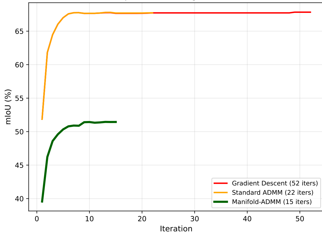
(d) Optimizer Convergence Curves
