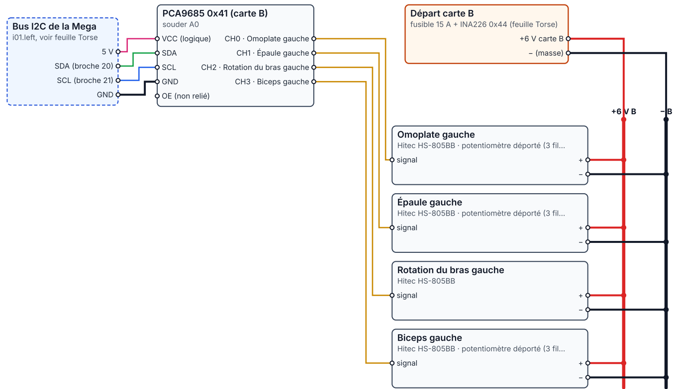
Carte B : bras et main gauche · PCA9685 0x41
