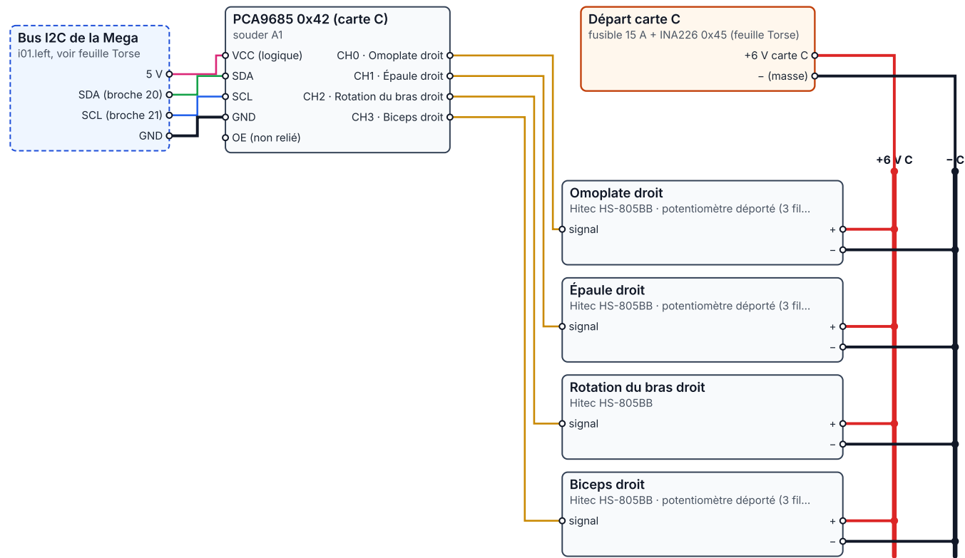
Carte C : bras et main droite · PCA9685 0x42
