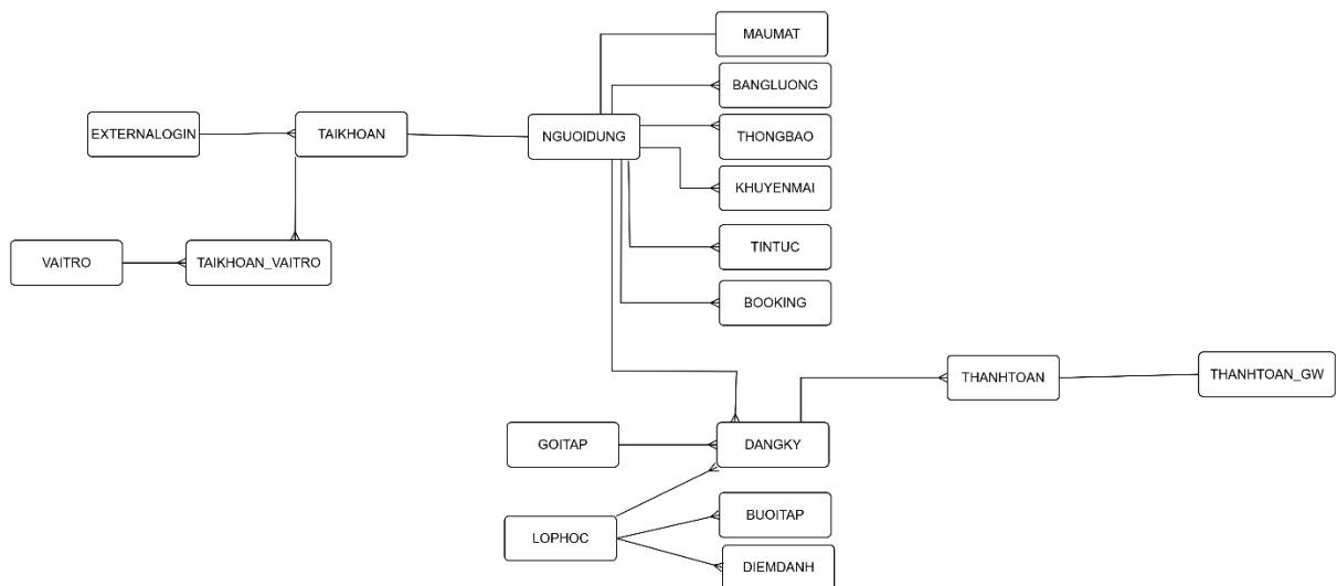
Hình 37: Lược đồ cơ sở dữ liệu của Website quản lý phòng Gym
