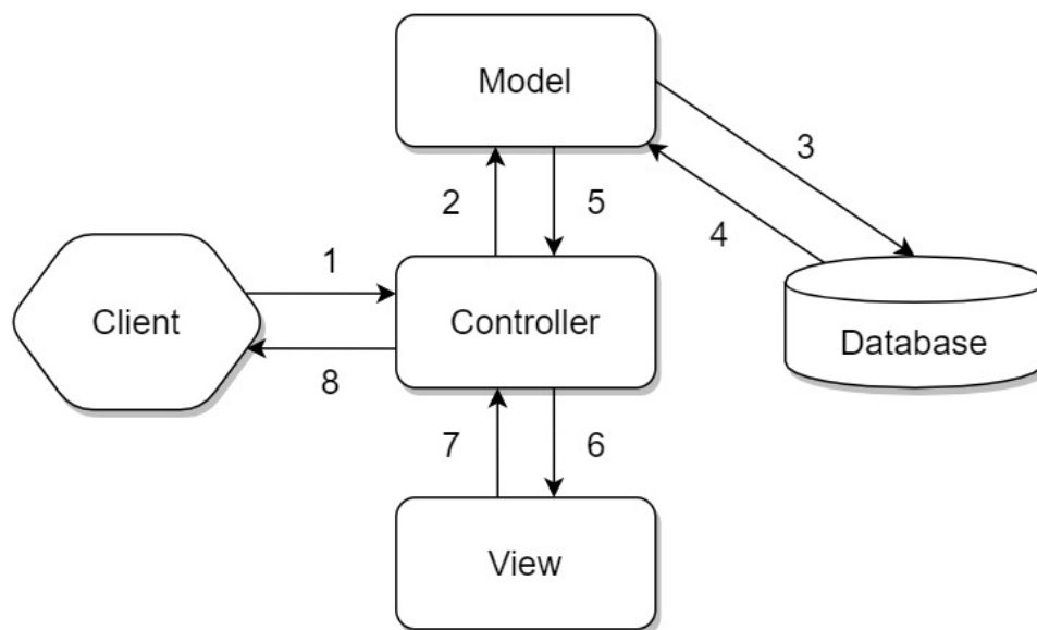
Hình 1: Luồng xử lý yêu cầu trong ASP.NET
