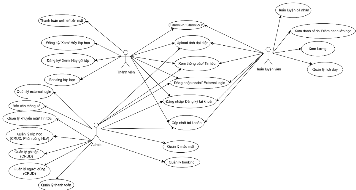
Hình 38: Sơ đồ Usecase Website quản lý phòng Gym
