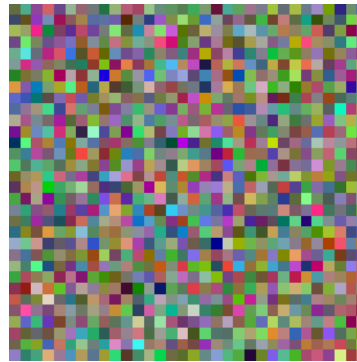
DP \sigma=1e-2
