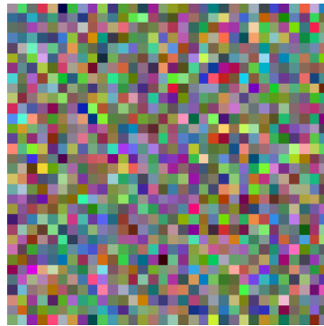
DP \sigma=1e-3
