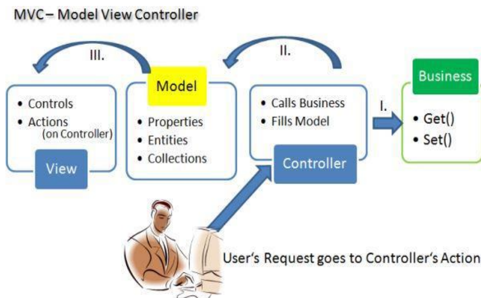
Hình 2: Các hoạt động của mô hình MVC.
