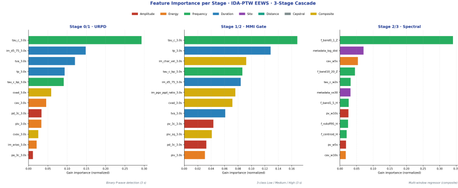
Fig. 3. Pentingnya fitur per-stage (gain ternormalisasi) untuk kaskade IDA-PTW yang dievaluasi di bawah CV 5-fold event-grouped. Kiri: Stage 0/1 URPD — deteksi gelombang-P biner pada jendela 3-s, didominasi oleh proxy frekuensi-sudut sumber \tau_c bersama deskriptor durasi ( t_p , t_{va} , t_{d5-75} ). Tengah: Stage 1/2 Gate MMI — routing tiga-kelas Rendah/Sedang/Tinggi pada jendela 3-s yang sama, di mana \tau_c tetap dominan tetapi sekarang informatif bersamaan dengan t_p , t_{va} , dan deskriptor intensitas komposit ( I_{char-vel} , rasio PGV/PGD, CVAD). Kanan: regresor spektral Stage 2/3 — komposit multi-jendela, didominasi oleh band frekuensi-rendah vertikal f_{band0-1\text{ Hz}, Z} bersama metadata site-path ( \log_{10}\Delta dan V_{S30} ) dan energi kumulatif CAV yang dikomputasi pada jendela 5-s.
