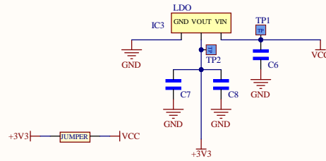
LDO 3V3
