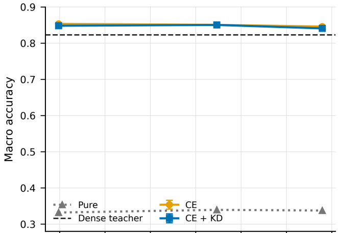
Llama-3.2-3B
