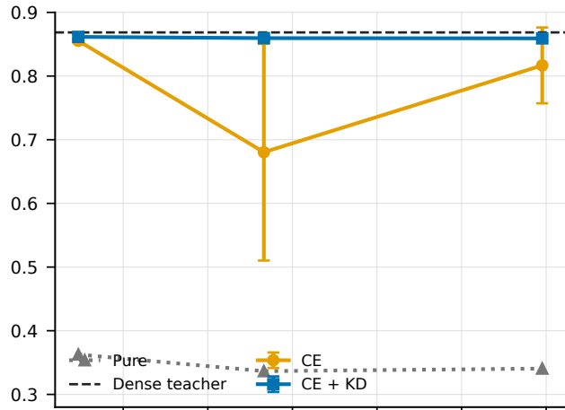
Llama-3.1-8B
