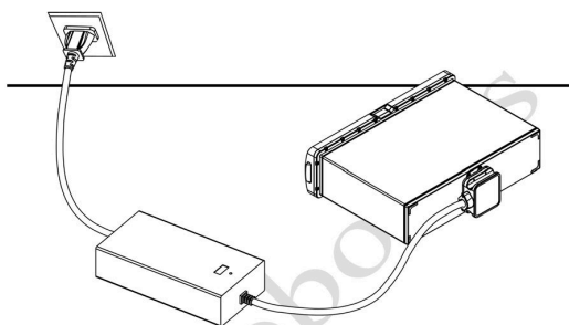
③ 连接 B2 电池
