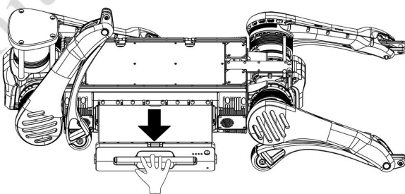
① 将电池从 B2 机身中取出 (向外拉出电池包提带)
