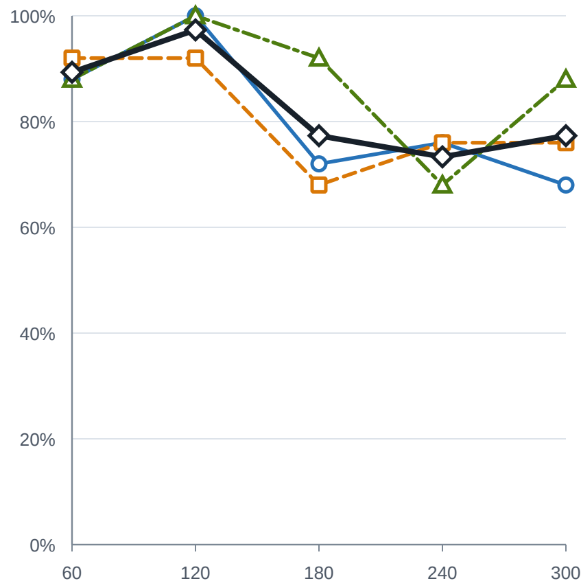
Claude Opus 5
