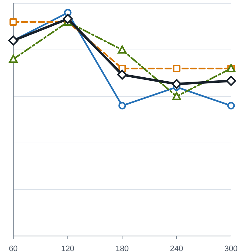
GPT-5.6 Sol
