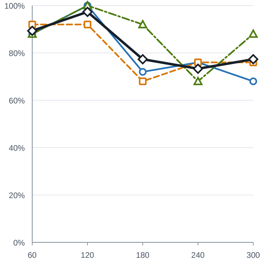
Claude Opus 5
