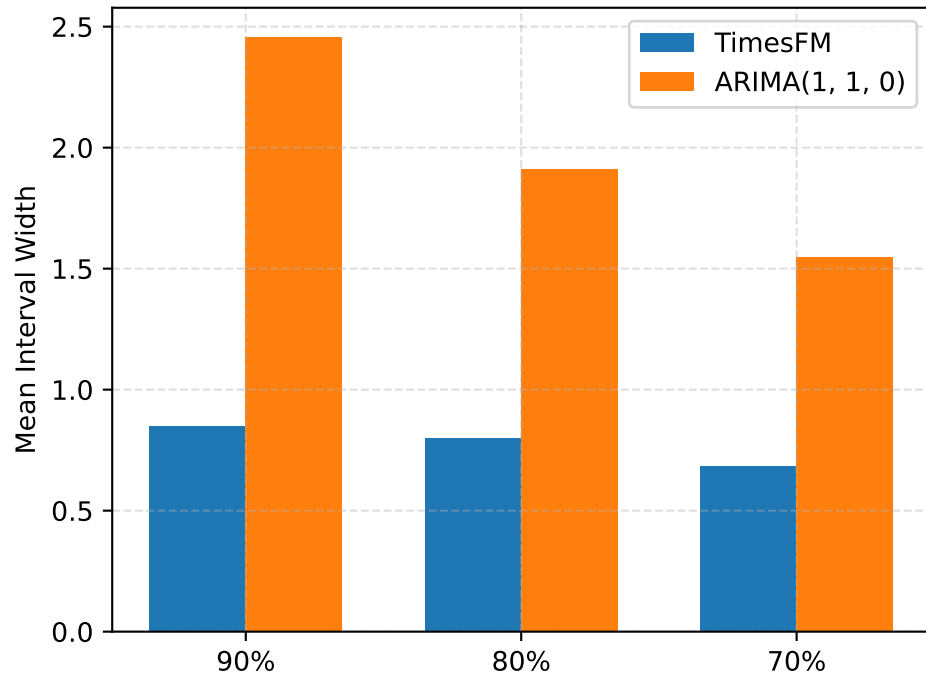
VERSIONED IL Width
