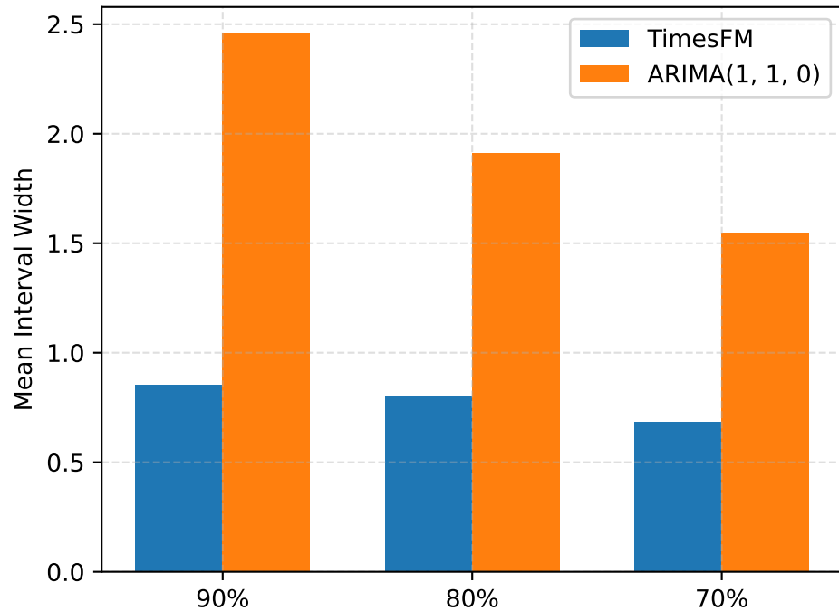
FINALIZED IL Width
