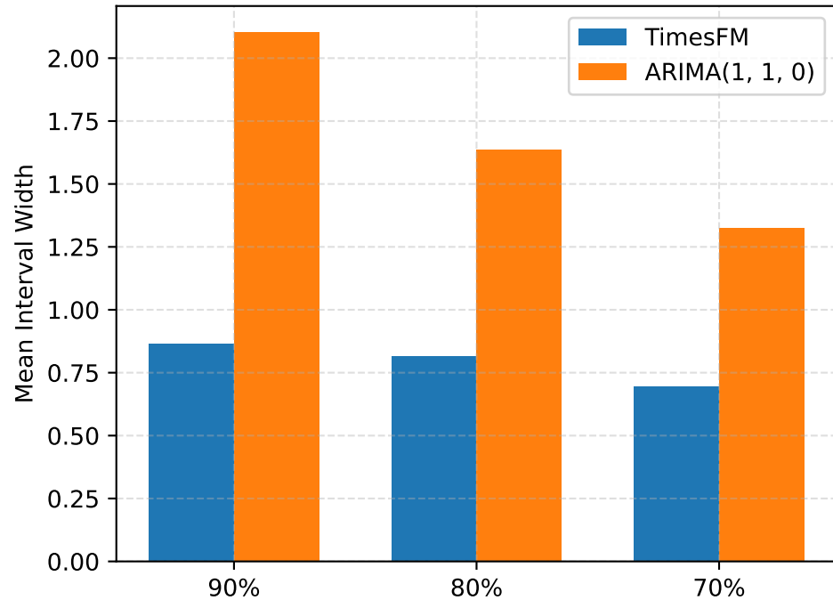
VERSIONED WI Width
