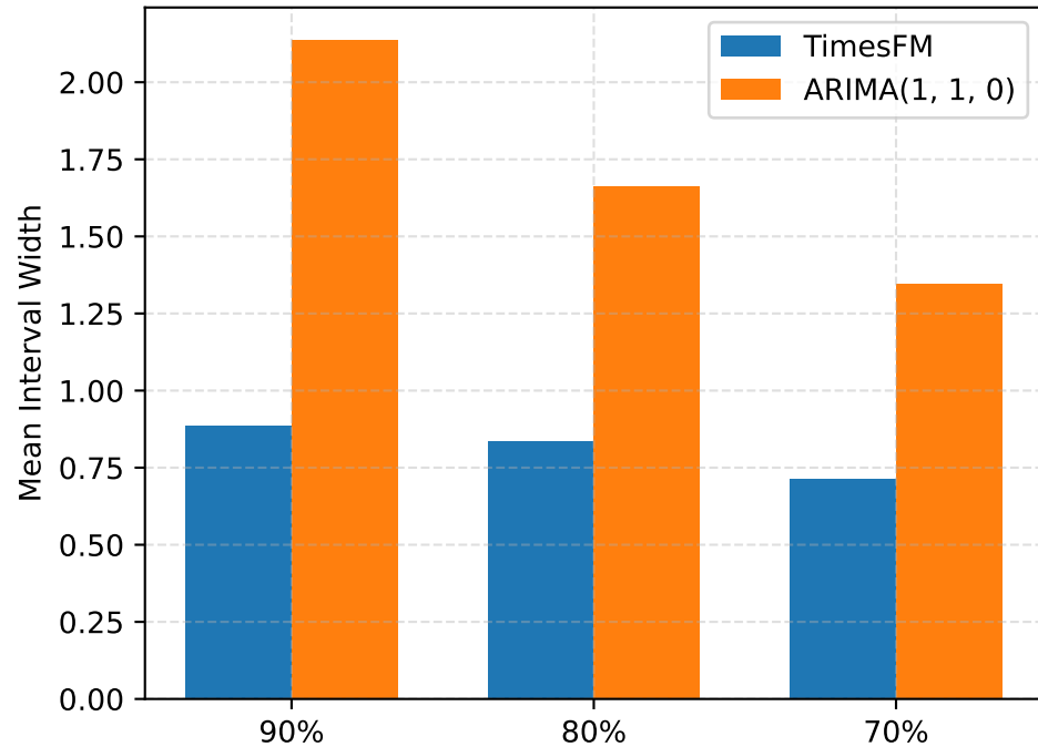
VERSIONED CA Width
