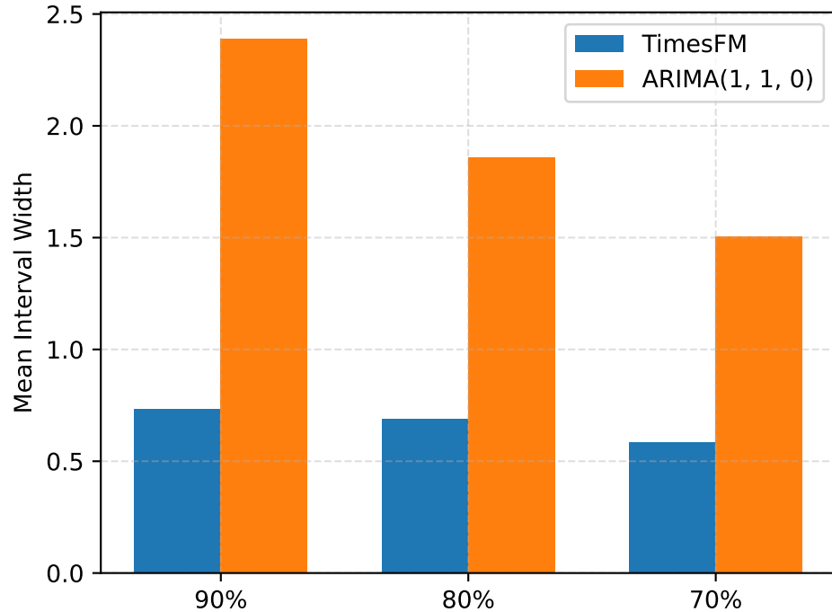
VERSIONED PA Width
