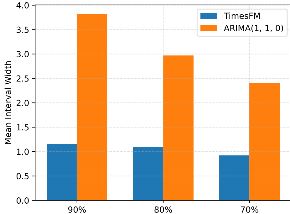
FINALIZED VA Width
