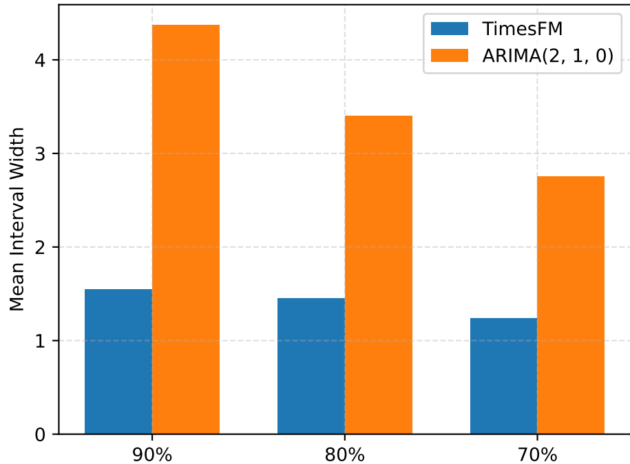
FINALIZED LA Width
