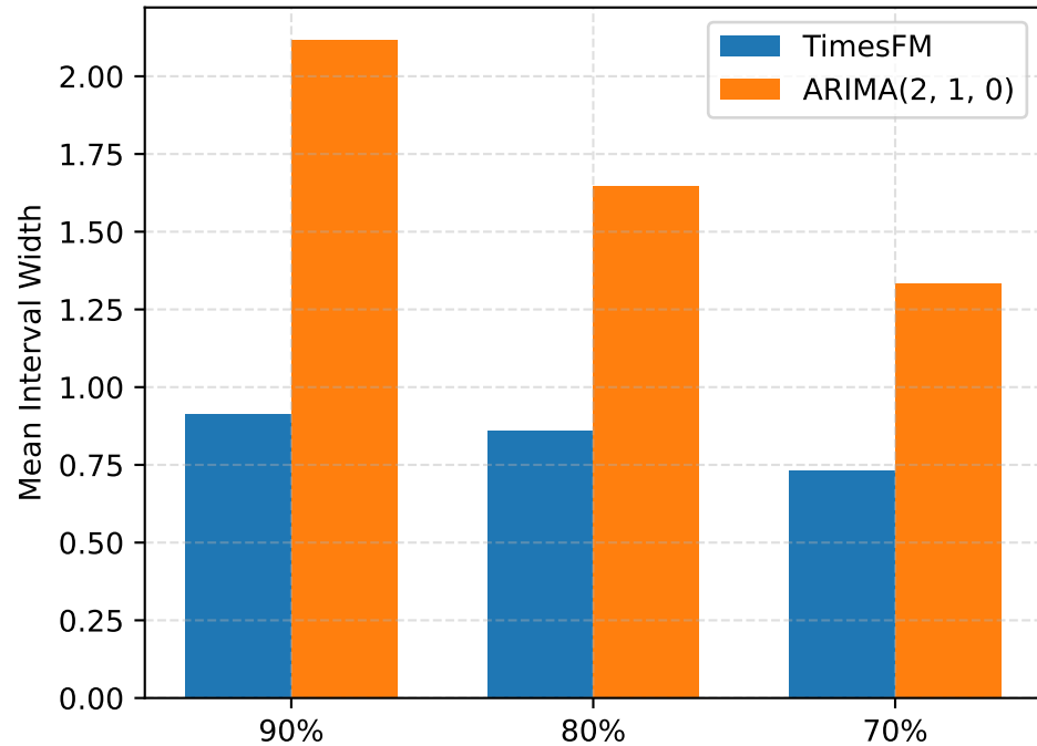
FINALIZED WI Width
