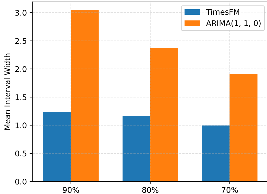
VERSIONED MN Width
