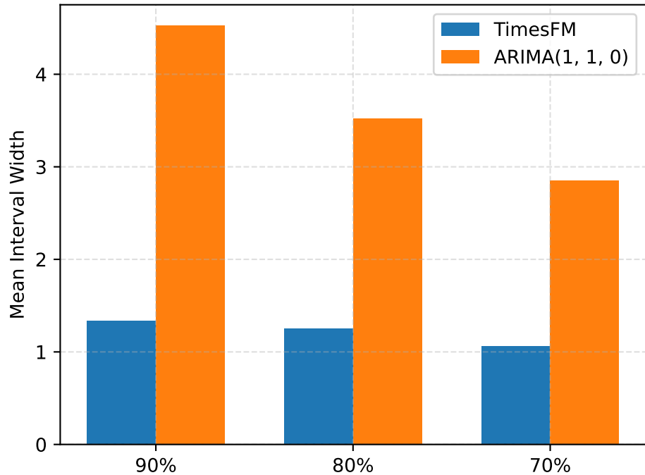
FINALIZED AL Width
