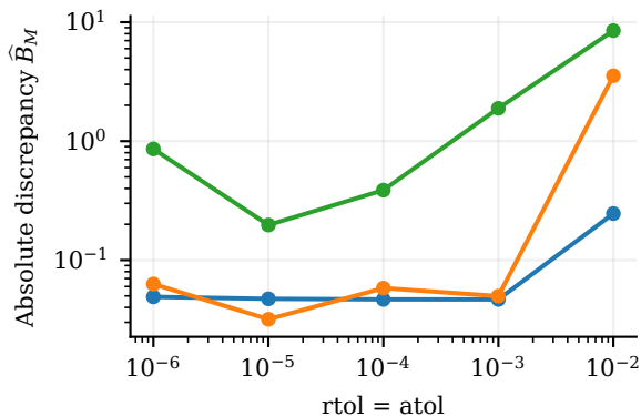
Rosenbrock — DOPRI5
