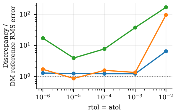
Rosenbrock — DOPRI5
