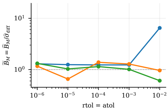
Rosenbrock — DOPRI5
