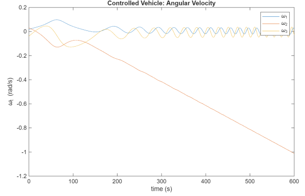
(d) \mathbf{u}_2 Applied: \omega_{B/N}
