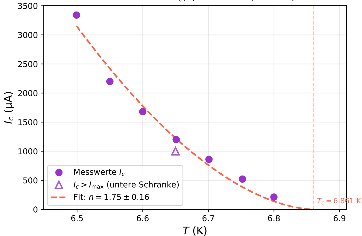
Kritischer Strom I_c(T) — Pb-Film (100 nm)
