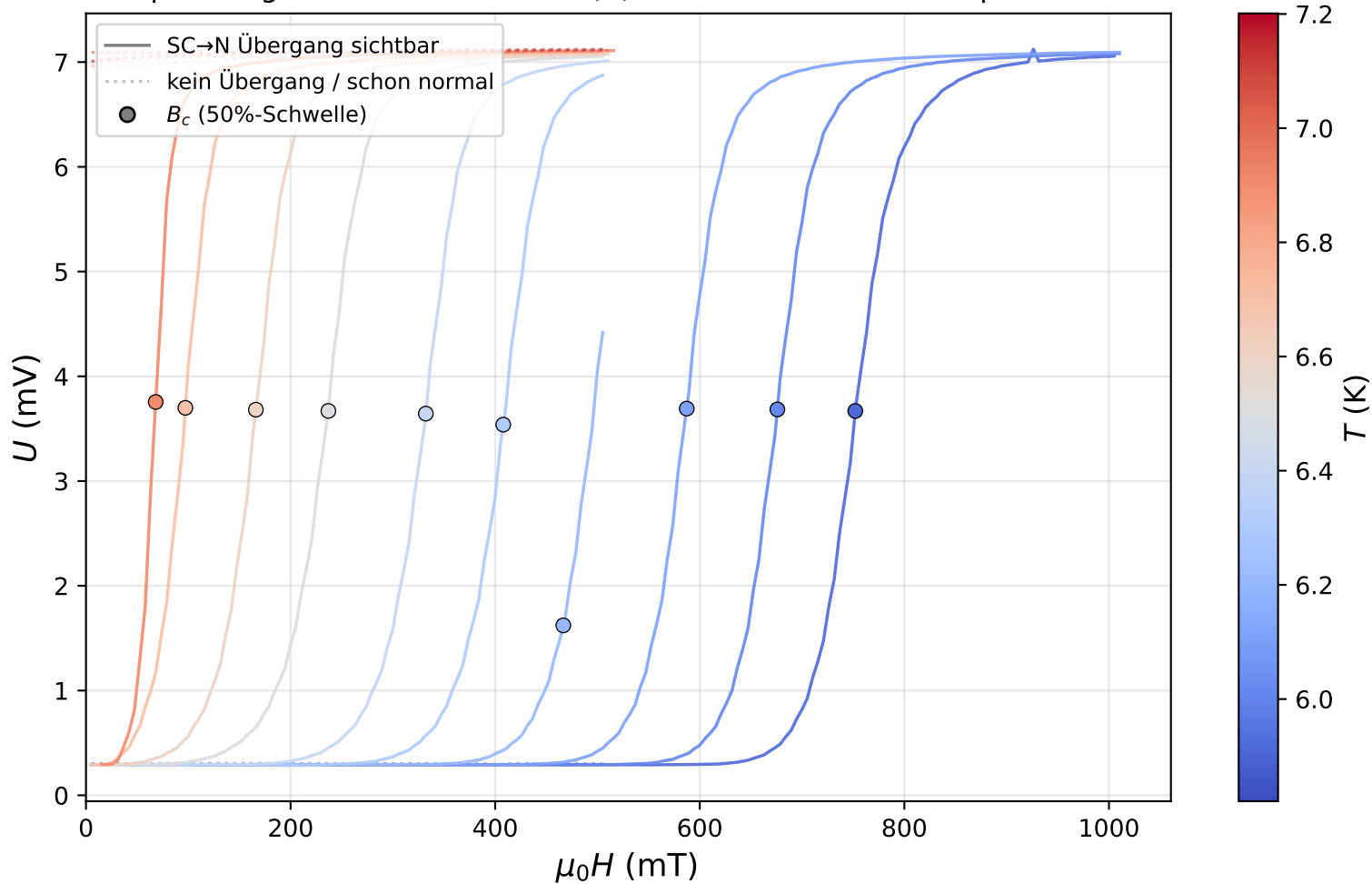
Spannungstransition Pb-Film: U(B) bei verschiedenen Temperaturen
