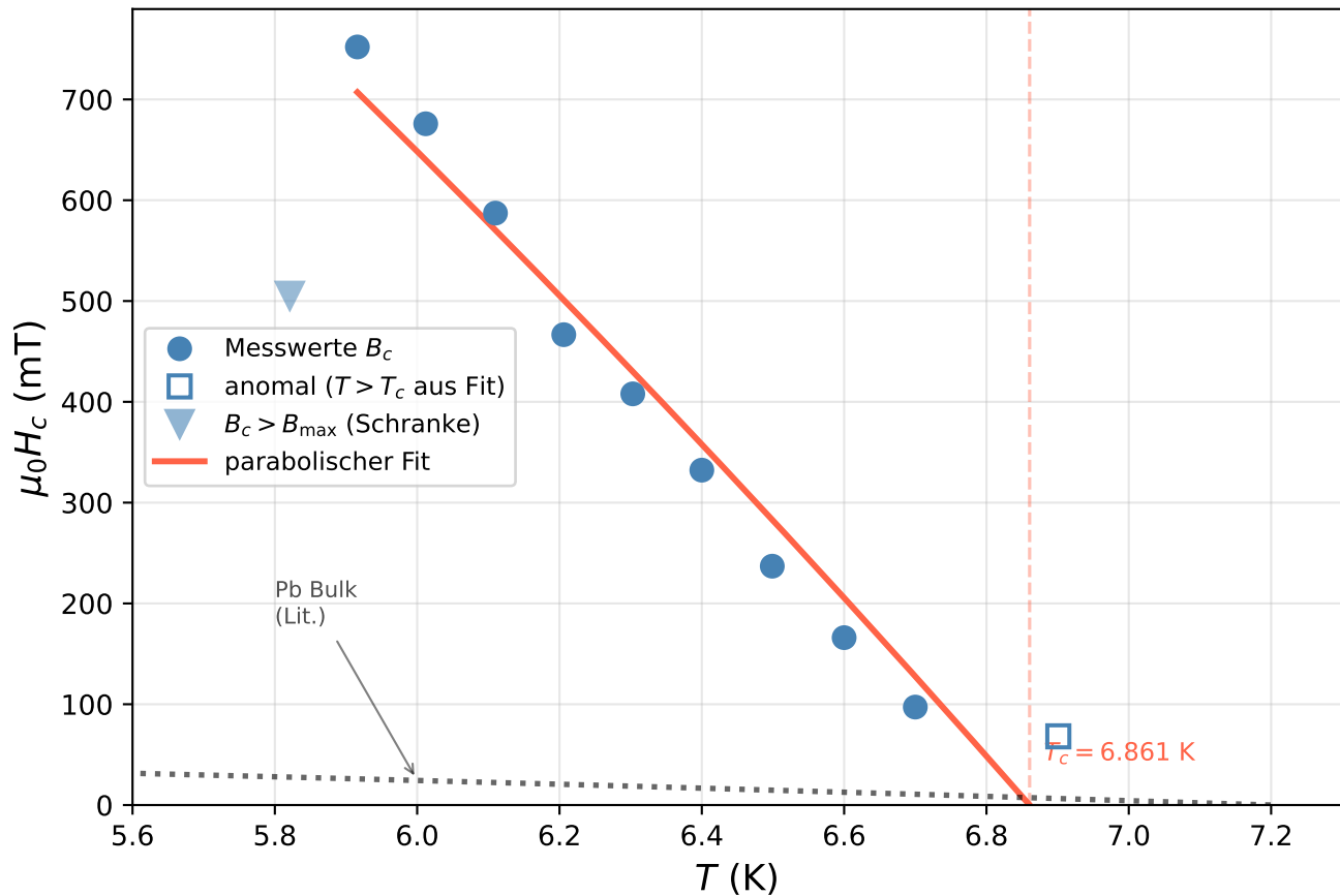
Phasendiagramm B_c(T) — Pb-Film (100 nm)
