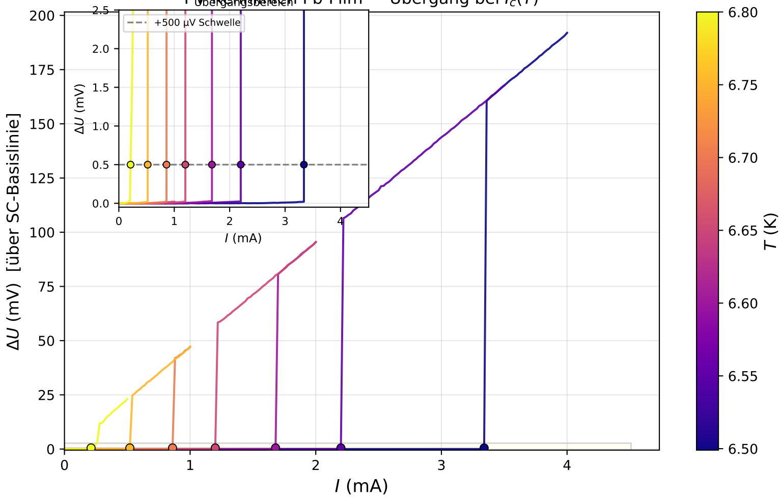
I-V Kennlinien Pb-Film — Übergang bei I_c(T)
