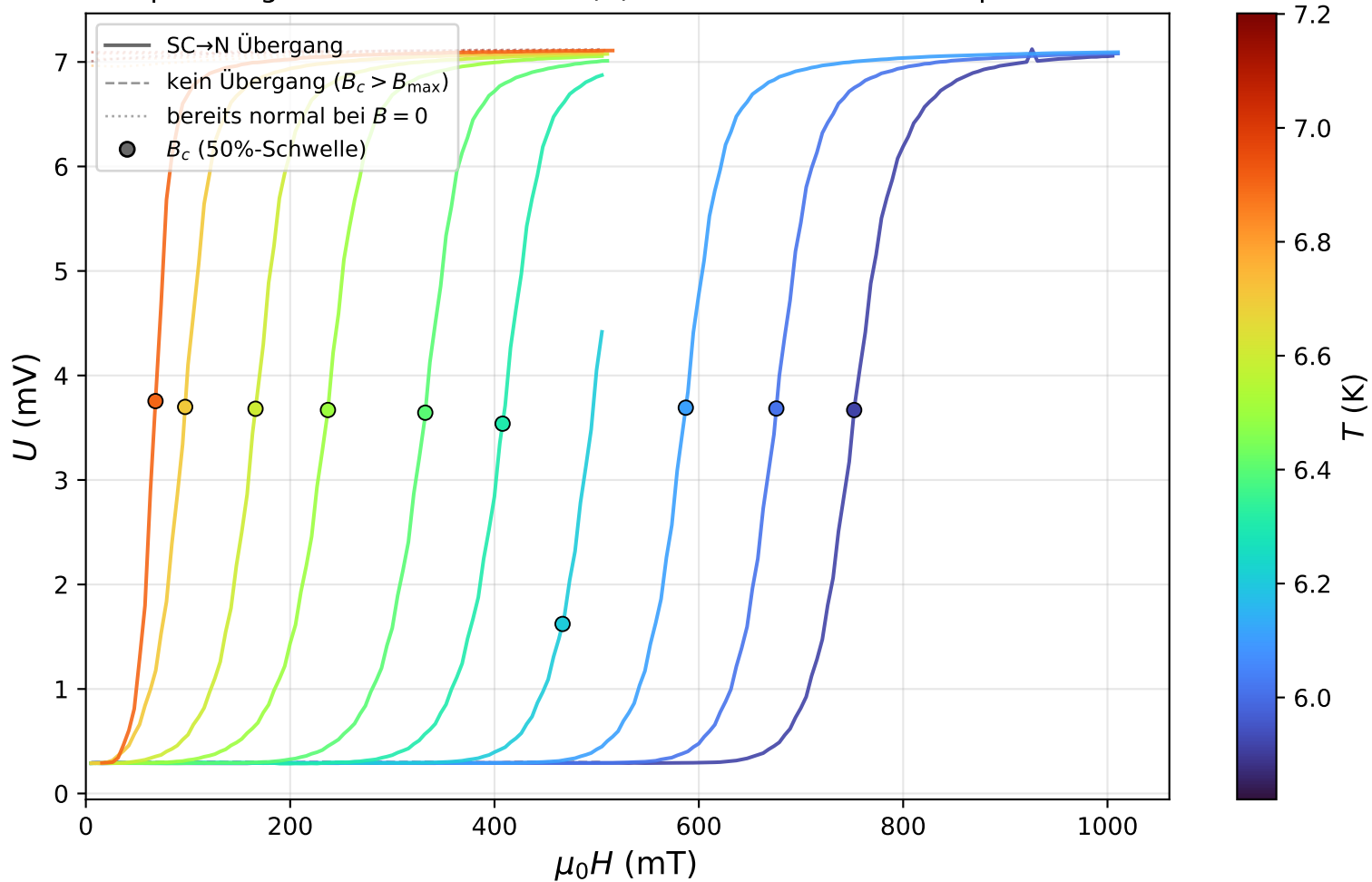
Spannungstransition Pb-Film: U(B) bei verschiedenen Temperaturen
