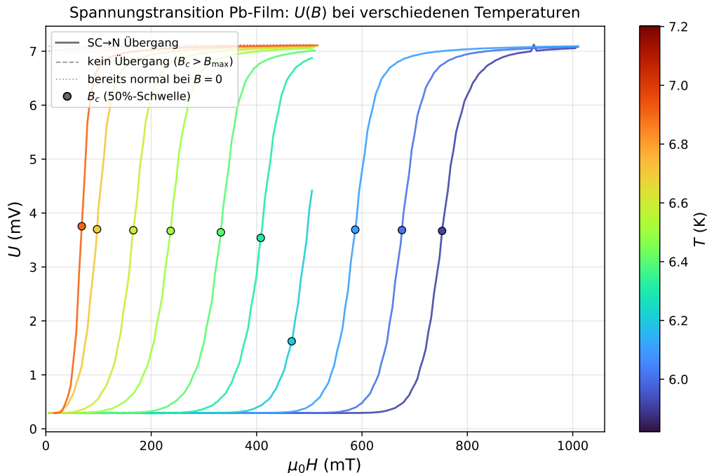
Abbildung 1: Spannungstransition U(B) des Bleifilms bei verschiedenen Temperaturen (Farbkodierung: blau = 5,82 K, rot = 7,20 K). Durchgehende Linien: klarer SC- \rightarrow N-Übergang. Gepunktete Linien: kein Übergang im Messbereich oder Film bereits normal bei B = 0 . Kreissymbole markieren die extrahierten B_c -Werte (50%-Schwelle).
