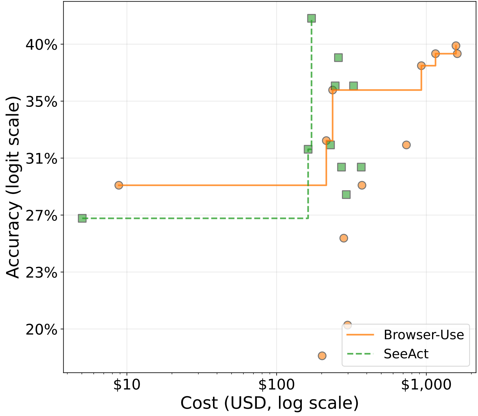
Online Mind2Web
