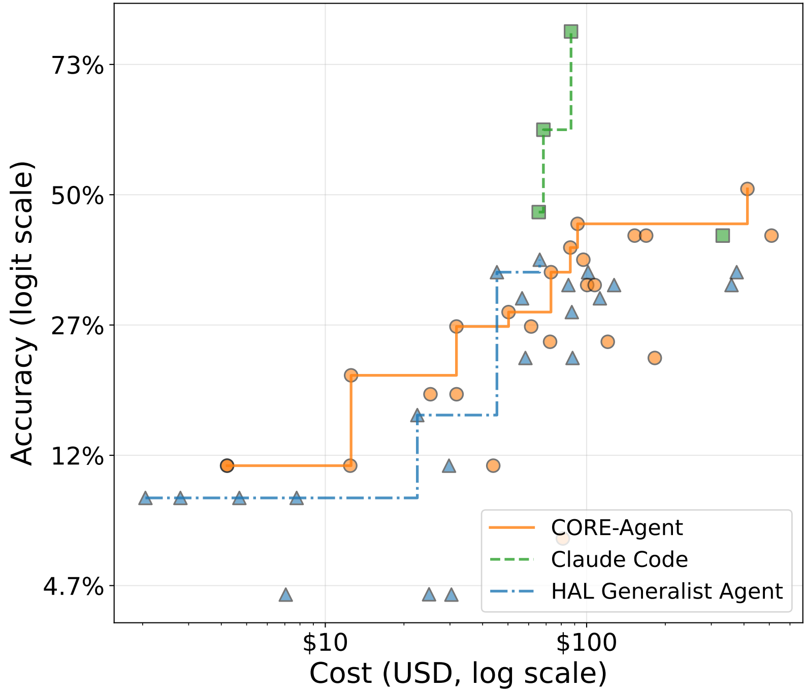
USACO
