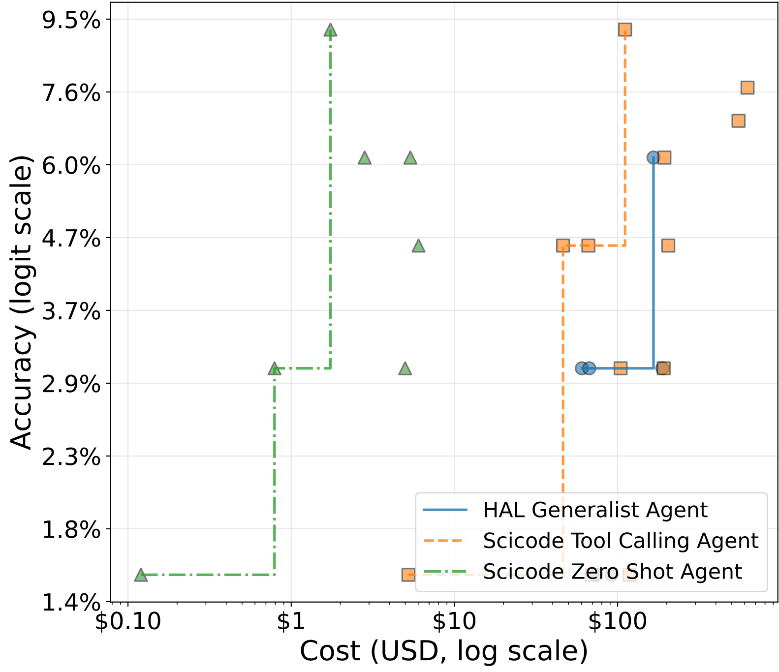
SciCode
